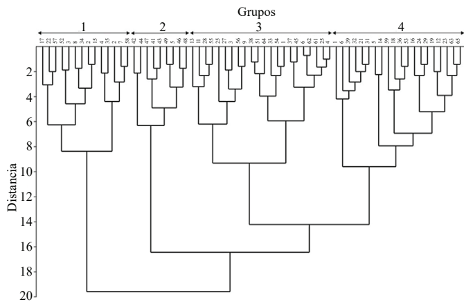
Figura 1. Dendrograma resultante del análisis de semejanza florística con las especies arbóreas encontradas en las parcelas de la UR Tzucacab 1.
